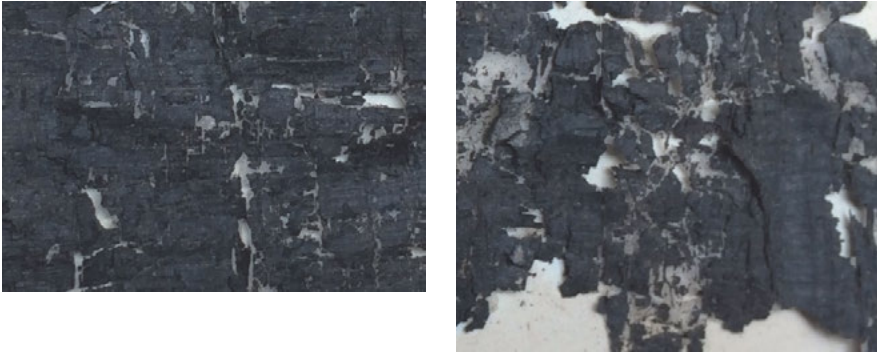
Abb. 20 und 21: Details eines Papyrus (PHerc. 1021) – Hügel und Risse (mit normaler Kamera).
