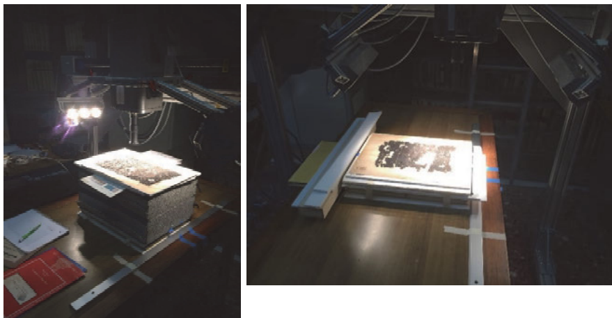
Abb. 30 und 31: Experimente 2018 mit Hyperspektraltechnik an PHerc. 1021 (Philodems Index Academicorum )
